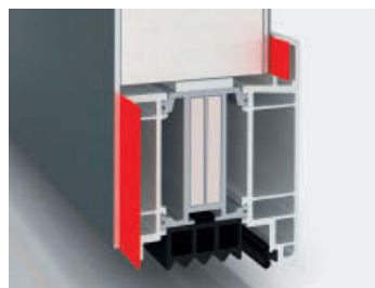
↑ Verklebung von Aufsatzfüllungen z. B.: tesa® ACXplus 7078
